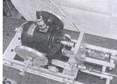
(a) (b) Hình 2. Một hệ tự di chuyển: (a) mô hình nguyên lý và (b) ảnh chụp thiết bị
