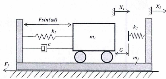
(a) (b) Hình 2. Một hệ tự di chuyển: (a) mô hình nguyên lý và (b) ảnh chụp thiết bị
